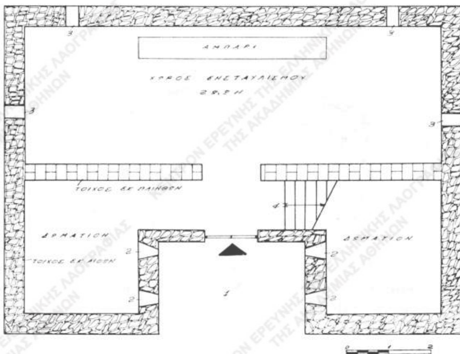
Σχ. 1. Κάτωφλις ἰσογείου οἰκίας οἰκογενείας Ἀραμπατζῆ. (Χωρεῖον Καρδιά).
