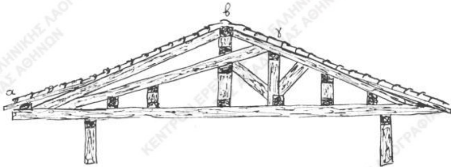
Σχ. 2. Κάθετος τομὴ στέγης μετὰ τὴν μεταξύ τῶν « γροιντιῶν » κρύπτην αβγ.
