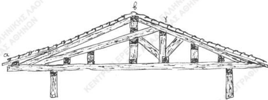
Σχ. 2. Κάθετος τομὴ στέγης μετὰ τὴν μεταξὺ τῶν « γροιντιῶν » κρύπτην ἀβγ.
