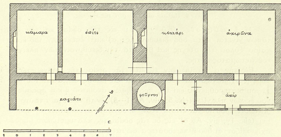
Εἰκ. 6. Κάτοπις παλαιᾶς οἰκίας χωρίου Δογαντζί τοῦ Διδυμοτείχου. (Γ. Μέγα, Θρακικαὶ Οικήσεις, εἰκ. 10).
