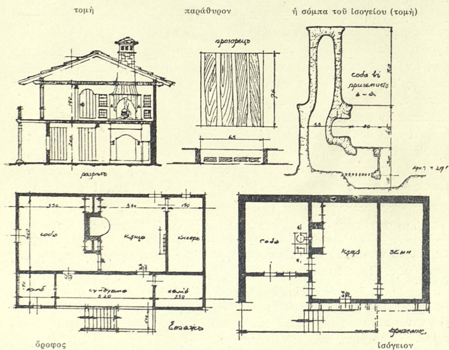
Είχ. 44. Κατόψεις και τομή της άνω οίκιας του χωρ. Μπούνοβο. (Zlatev, Balg. kasta ειχ. 56)
