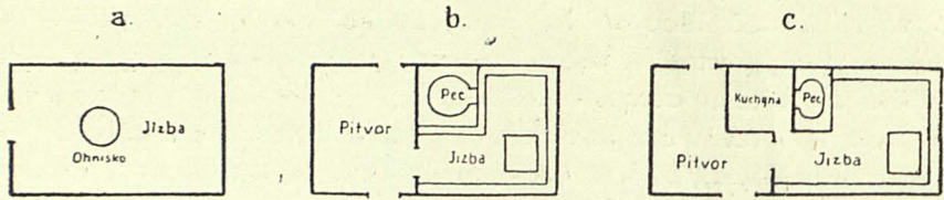
Εἰκ. 45. Τρεῖς ἐξελικτικαὶ μορφαὶ σλοβακικῆς οἰκίας εἰς τὰ δυτικὰ Καρπάθια: jizba=δωμάτιον, ognisko=ἔστια, pitvor=προθάλαμος, pec=θερμάστρα, kuchnja=μαγειρεῖον (L. Niederle, Manuel de l'antiquité slave 2, 107).
