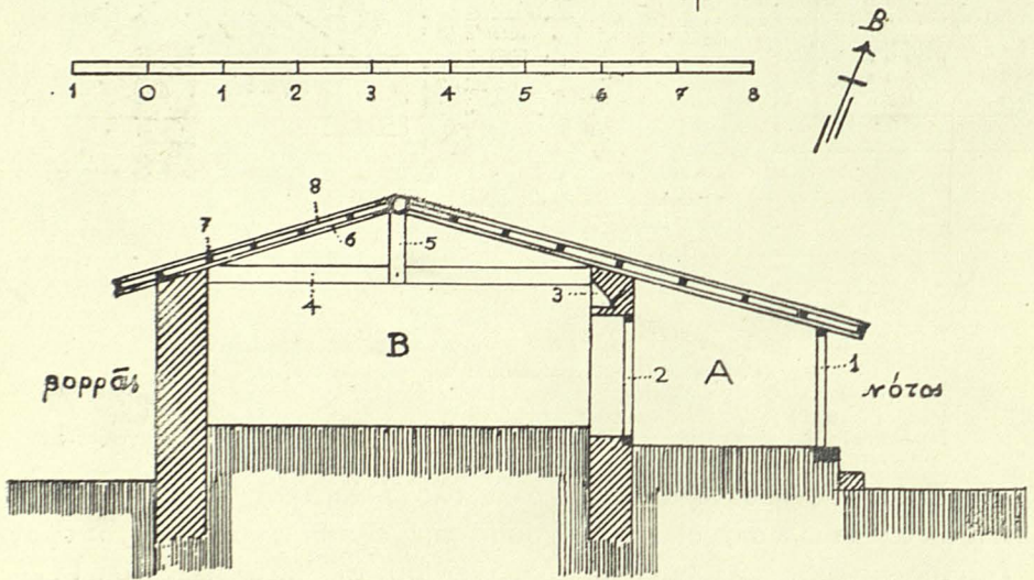
Εικ. 3. Κάτοψις και κατά πλάτος τομή παλαιᾶς οἰκίας τοῦ χωρίου Τριφύλλι.
