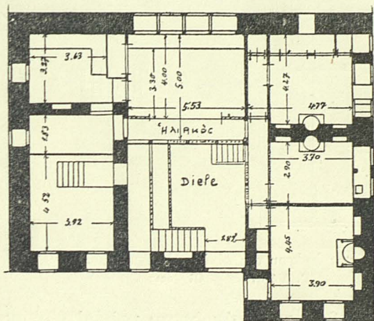
Εἰκ. 24. Κάτοψις ἀρχοντικοῦ τῆς Σιατίστης. (Ἄριστ. Ζάχος, ἐνθ' ἂν. σ. 248. Βλ. Γ. Μέγα, Θεσσ. Οἰκ. εἰκ. 91)
