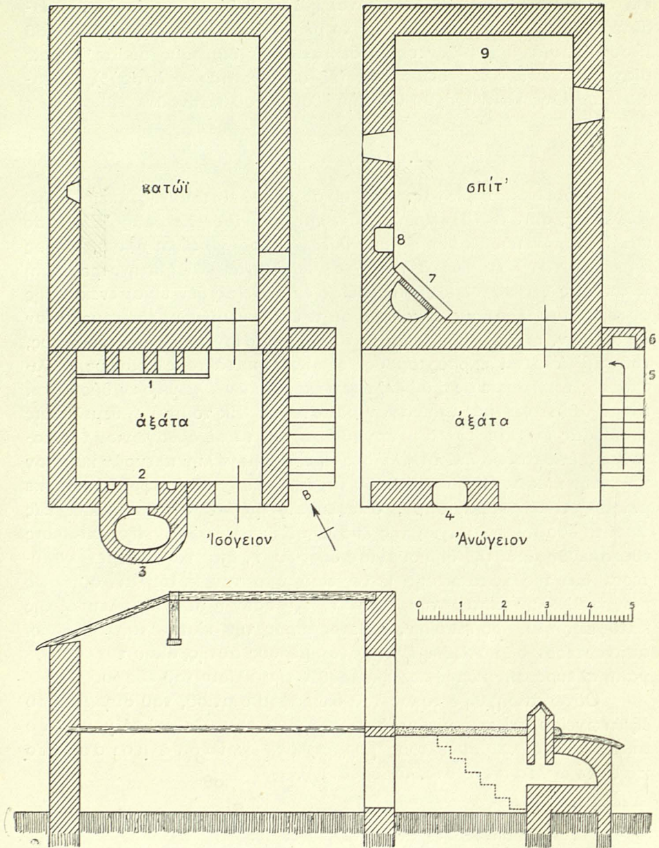
Εἰξ. 13. Κάτοπις καὶ κατὰ πλάτος τομὴ σπιτιοῦ τοῦ χωρίου Ἁγ. Σοφίας τῆς Λήμνου.
