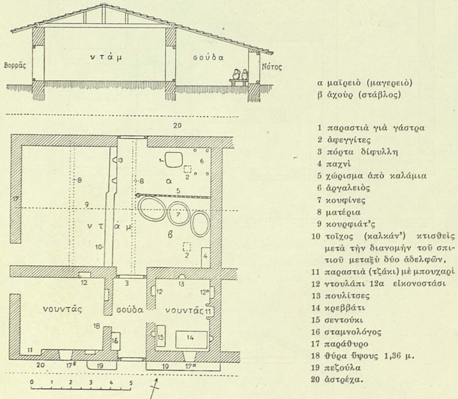
Εἰκ. 9. Κάτοψις καὶ κατὰ πλάτος τομὴ παλαιοῦ σπιτιοῦ τῶν Σοφάδων. (Γ. Μέγα, Θεσσαλικαὶ οἰκῆσεις, εἰκ. 11)
