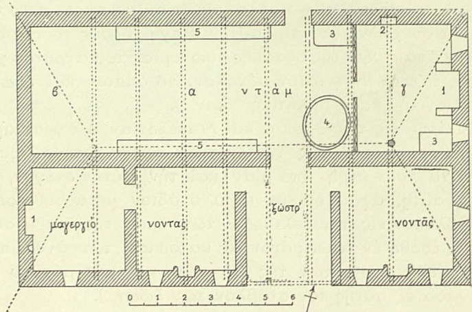
Εἰκ. 10. Κάτοψις σπιτιοῦ μὲ τὸ προστώφ ἐνσωματωμένον εἰς τὴν οἰκοδομὴν.
