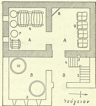
Εἰκ. 18. Κάτοψις οἰκίας Ἁγίου Ἀχακίου
